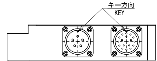
C矢視図 VIEW C
