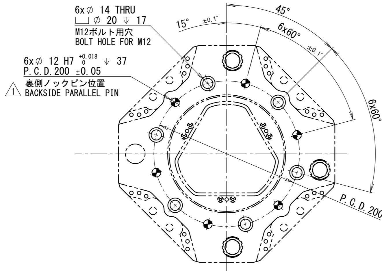
矢視図 A: 取合い寸法図 VIEW A: CONNECTING DIMENSION VIEW
