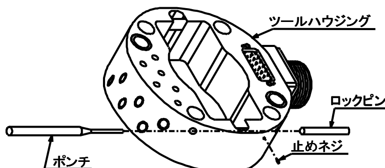
図18. ロックピンの交換
