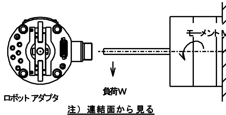
図5. ATCの取付方向
