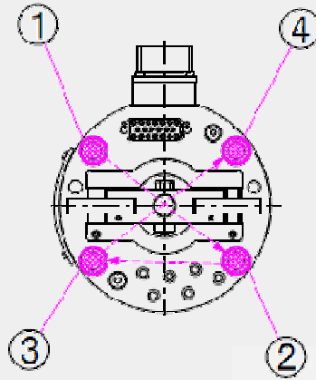
ボルトの締め付け順序及び注意事項
