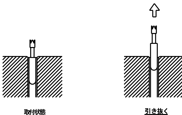
図13. ツール側スプリングピンの交換
