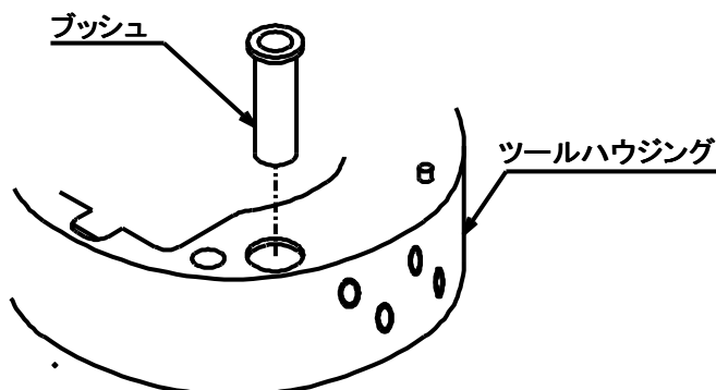
図17. ブッシュの交換
