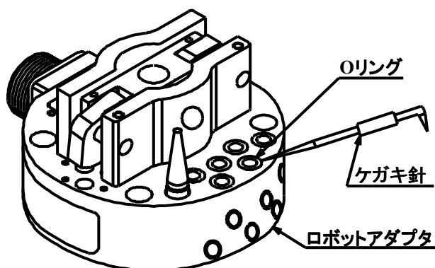
図15. Oリングの交換
