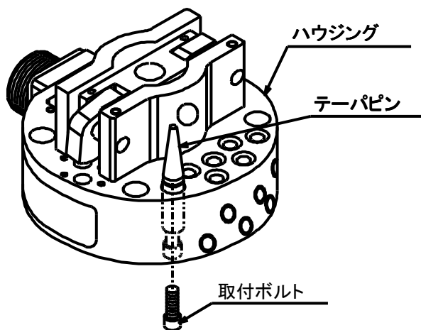
図16. テーパーピンの交換
