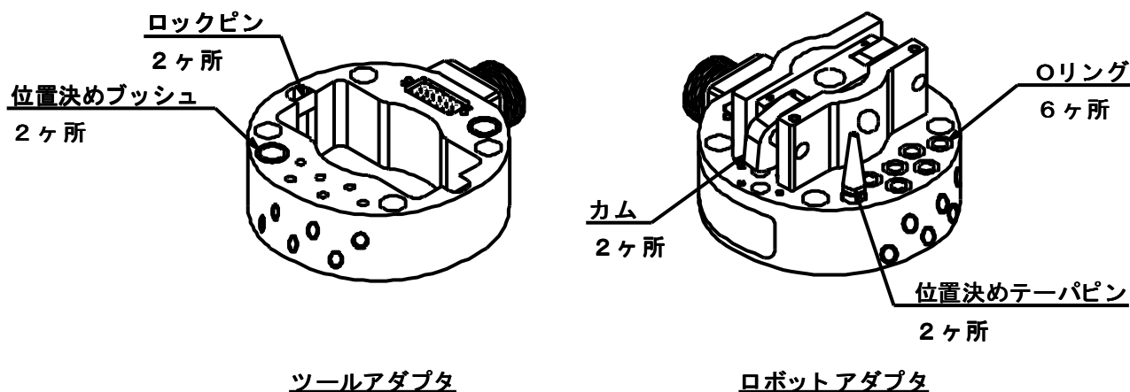
図12. ATC給脂箇所
