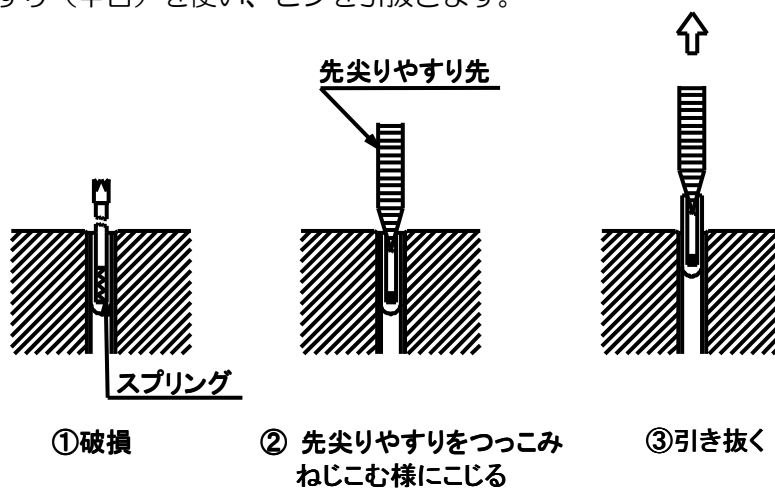
図14. 折損ピンの引き抜き
