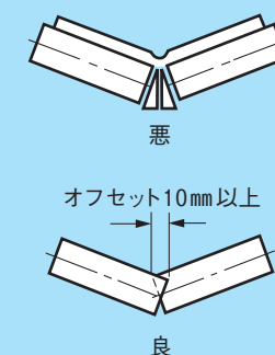
図-28 2本ローラトラフ
